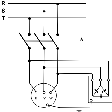
Doğrudan doğruya şebekeye bağlanan kısıdevreye rotorlu bir asenkron motorun bireysel kompanzasyonu
